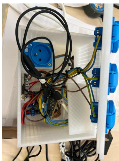
Obrázok 34 Vnútny obsah riadiacej jednotky Zdroj: Bc. Daniel Trst'án
