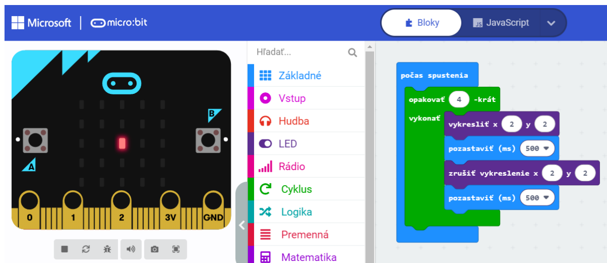
Obrázok 1 Príkaz "opakovať 4 krát"
