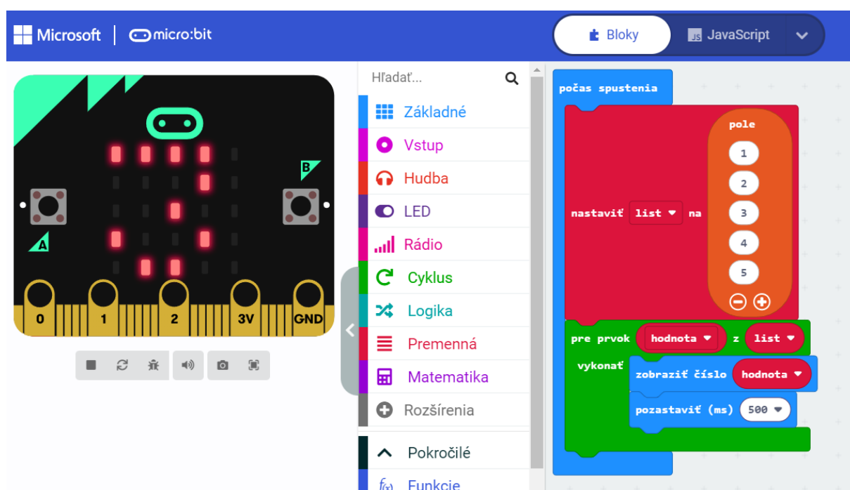
Obrázok 4 Príkaz "pre prvok hodnota z list"
