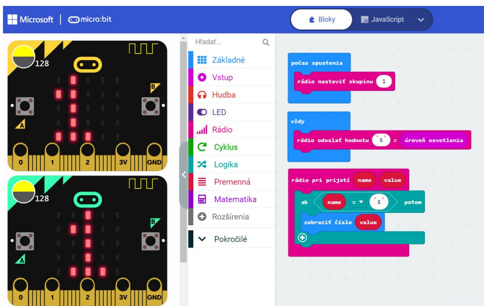
Obrázok 6 Príkaz "rádio pri prijatí name value"
