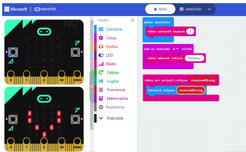
Obrázok 4 Príkaz "rádio odoslať reťazec"
