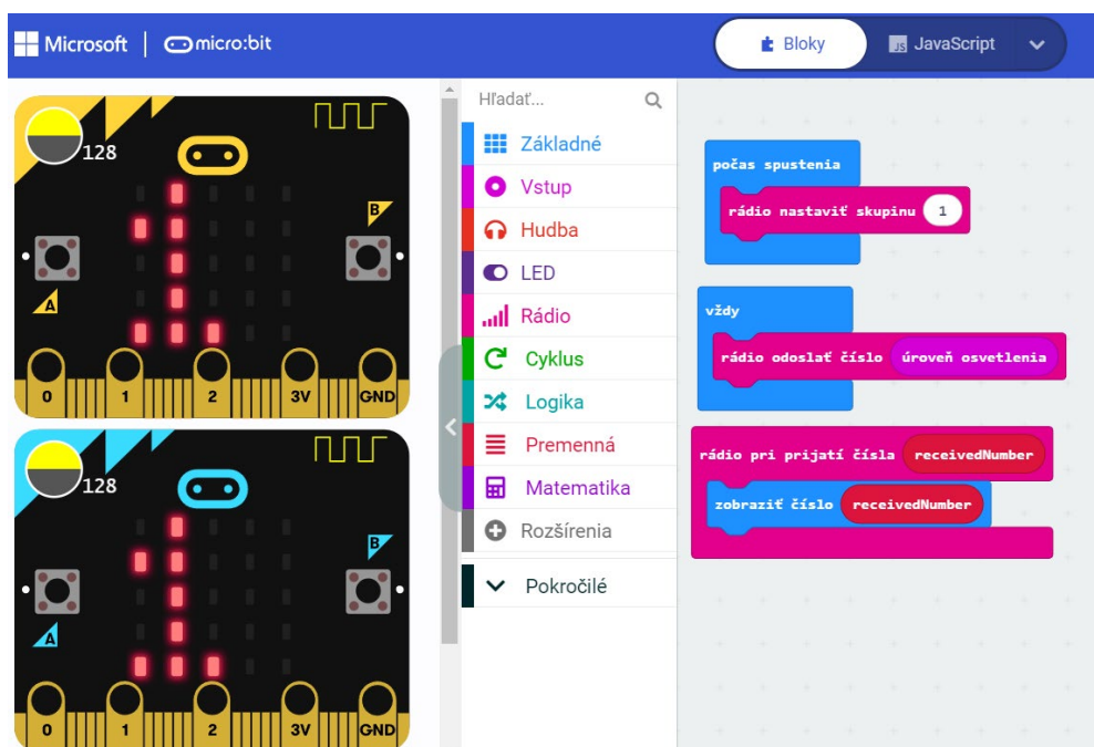
Obrázok 5 Príkaz "rádio pri prijatí čísla"
