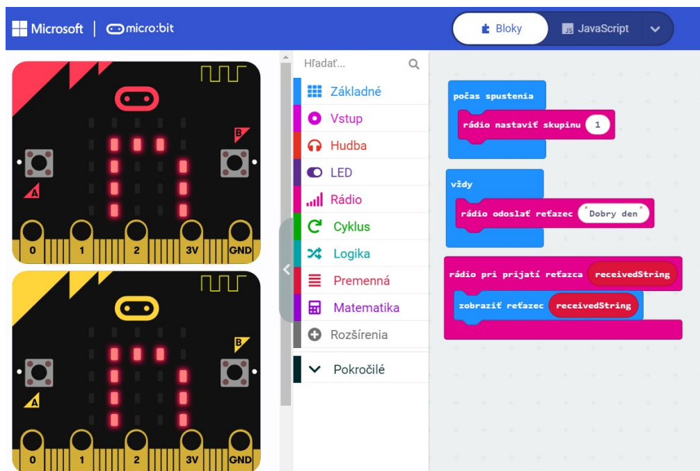
Obrázok 7 Príkaz "rádio pri prijatí reťazca receiveString"
