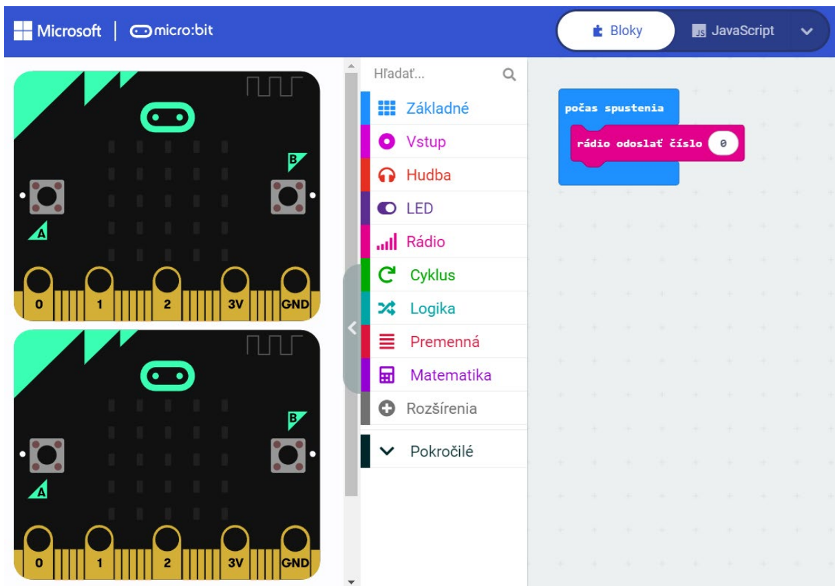
Obrázok 2 Príkaz "rádio odoslať číslo 0"
